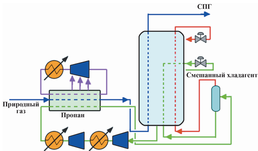
Рис. 3. Принципиальная технологическая схема процесса C 3 MR [5]
