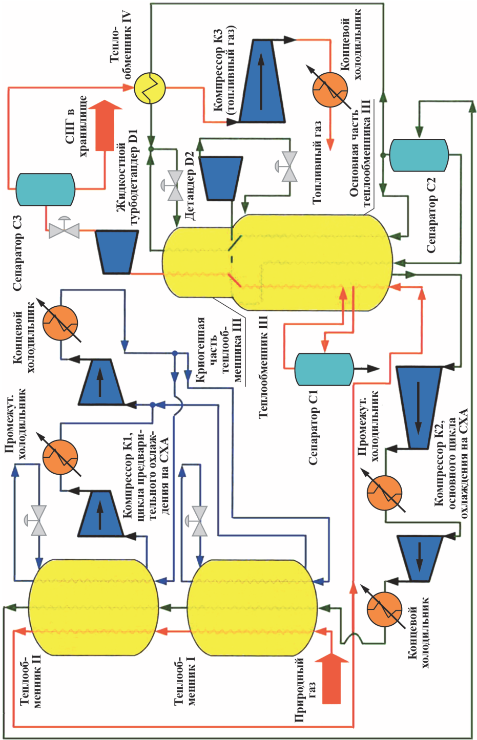
Рис. 5. Принципиальная технологическая схема процесса DMR [6]
